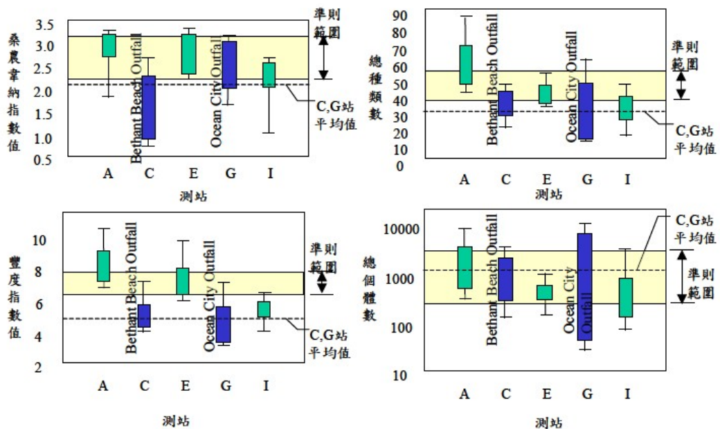
圖 3-2 污水放流管生物準則比對 (範例)
